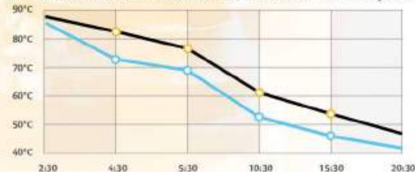
Tenuta del calore a 20 min. dalla cottura / Heat retention level 20 min. after cooking
